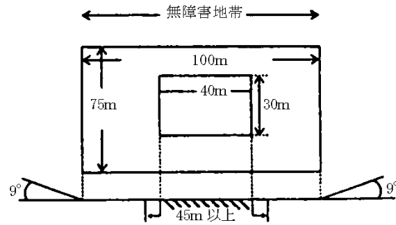
図3 ヘリポート
