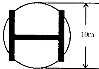
図3 ヘリポート
