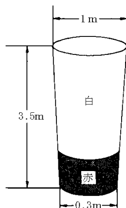
図1 吹流し
